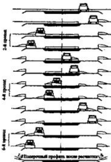
Рис. 15. Схема проходов снегоочистителей при расчистке дороги, занесенной толстым слоем снега (при отсутствии роторных снегоочистителей)
