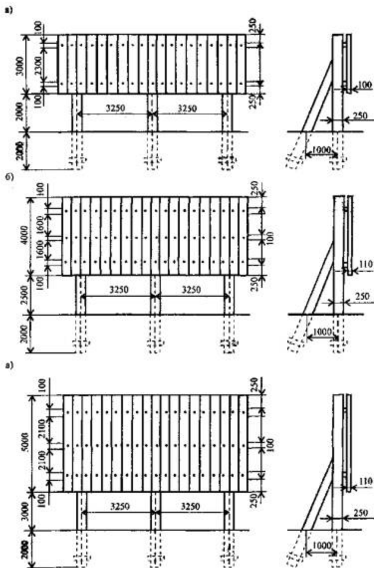
Рис. 7. Снегопередающие деревянные заборы (размеры даны в мм)
