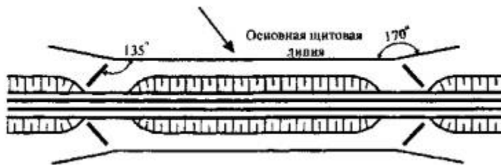
Рис. 11. Ограждение мест перехода из выемки в насыпь
