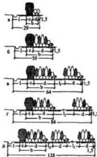
Рис. 4. Типовые схемы усиления существующих снегозащитных лесных насаждений вдоль автомобильных дорог при объеме снегоприноса ( m^3/m ):
