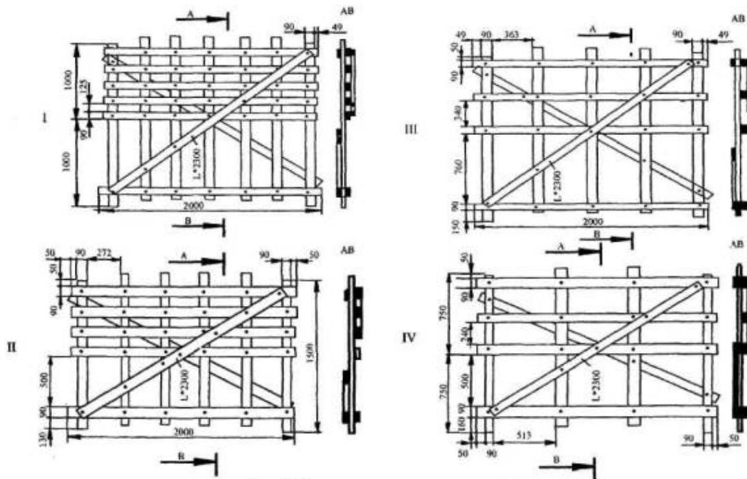
Рис. 9. Переносные решетчатые щиты (размеры даны в мм)
