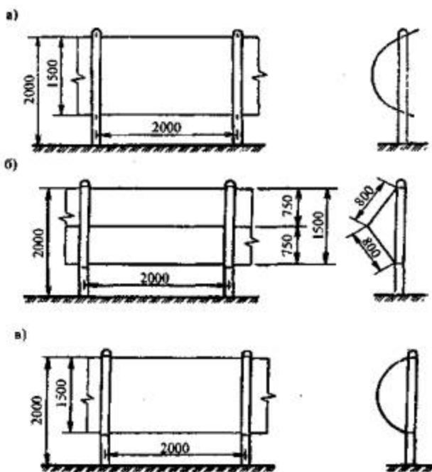
Рис. 12. Временные пространственные снегозащитные средства (ВПС):
