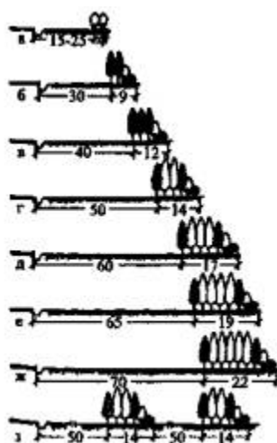
Рис. 2. Типовые схемы снегозащитных лесных насаждений вдоль автомобильных дорог при объеме снегопереноса ( m^3/m ):
