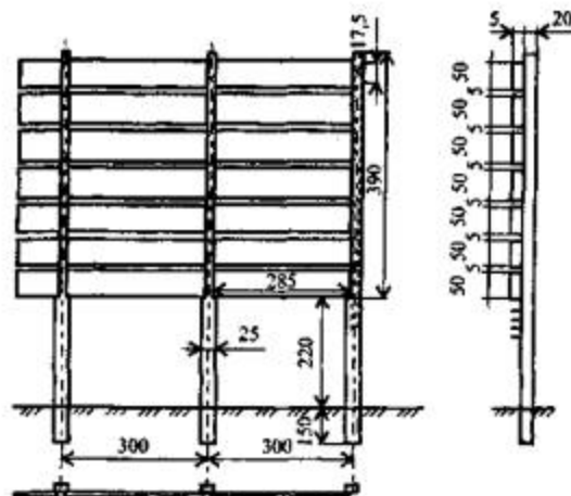
Рис. 8. Снегопередающая керамзитобетонная перегородка (размеры даны в см)
