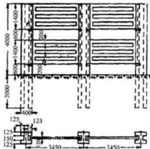
Рис. 6. Железобетонный снегозадерживающий забор (размеры даны в мм)
