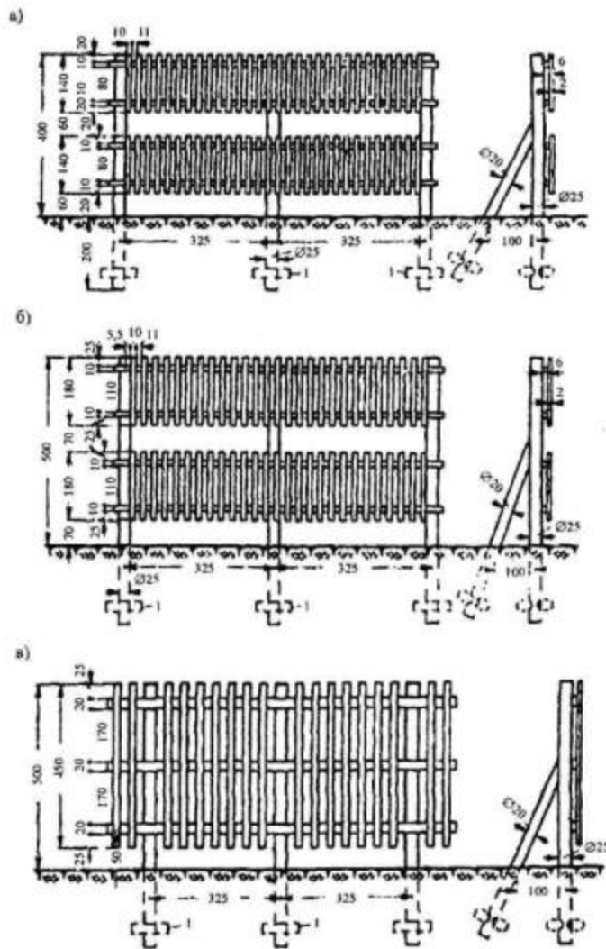
Рис. 5. Рекомендуемые типы снегозадерживающих заборов:
