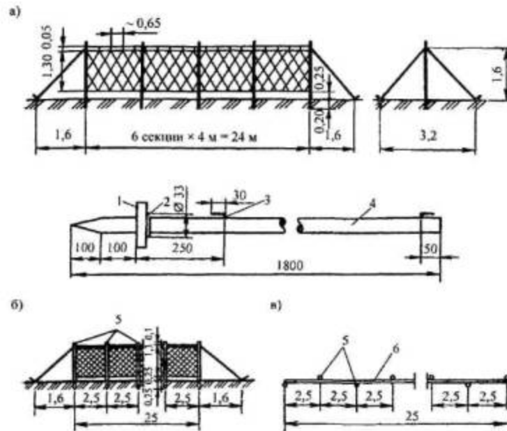
Рис. 13. Снегозадерживающие полиэтиленовые сетки:
